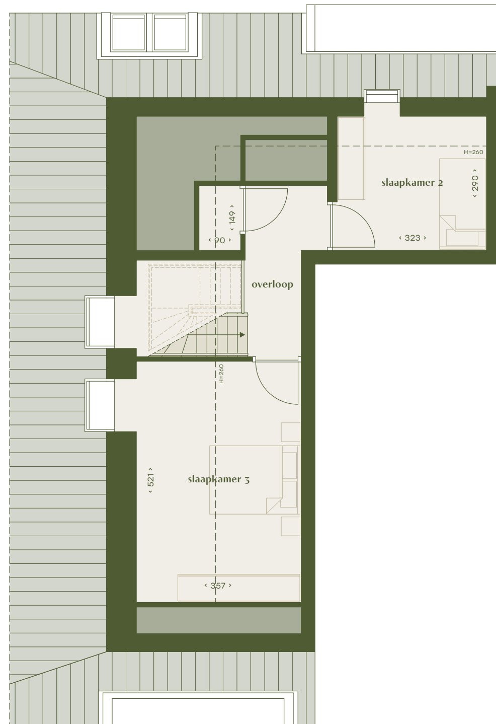
Plattegrond maisonnette type C - verdieping 4
