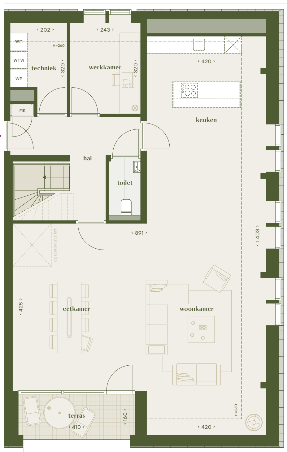
Plattegrond maisonnette type E - verdieping 3 - optionele indeling
