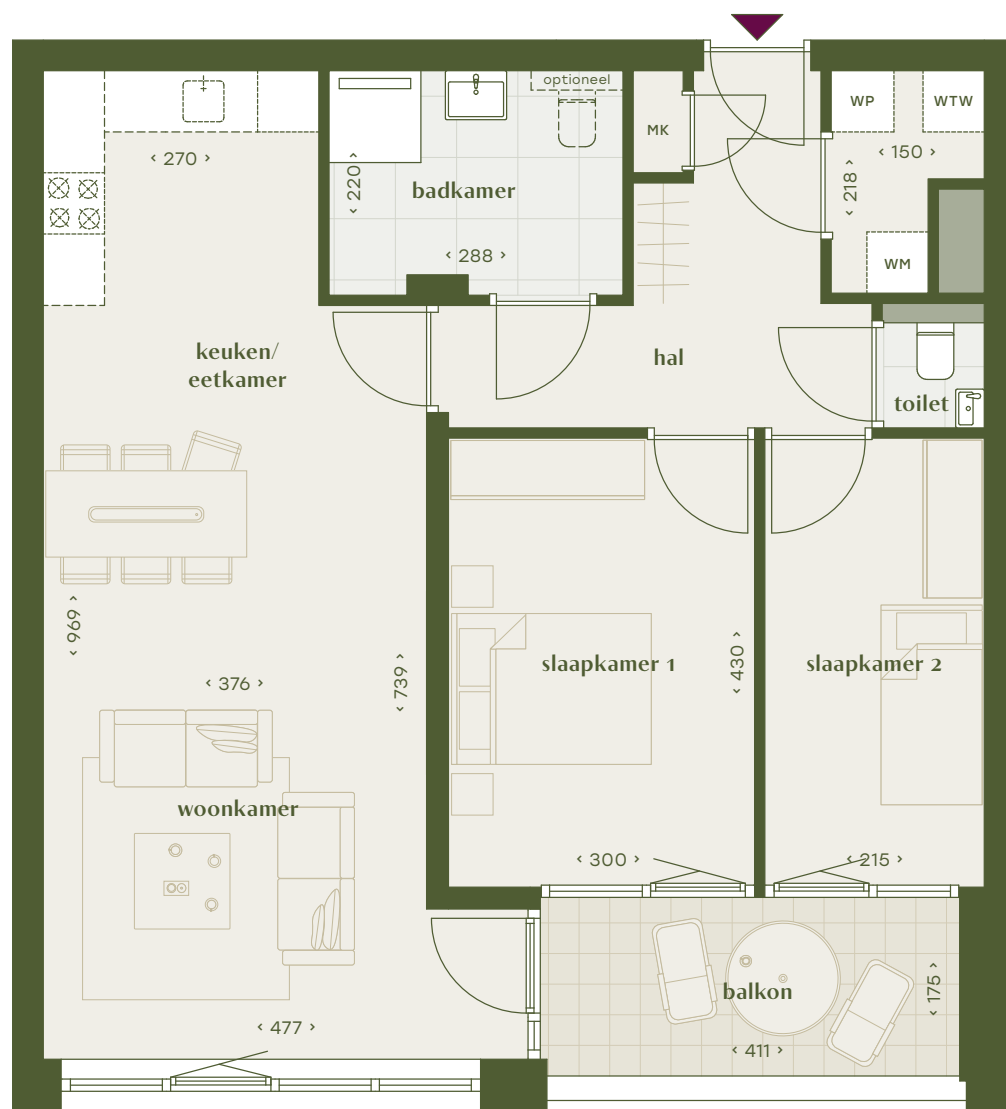
Plattegrond appartement type B
